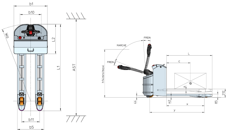
EP 20 Inox Premium - Disegno quotato
