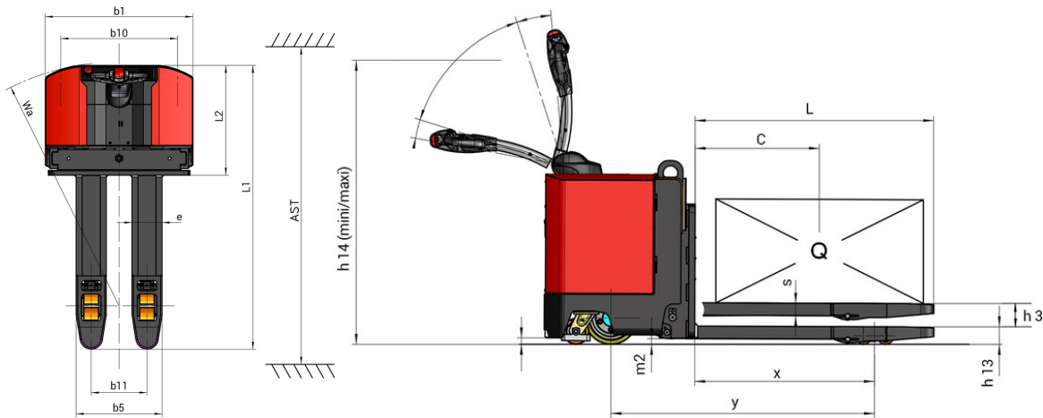
EP 730 - Disegno quotato
