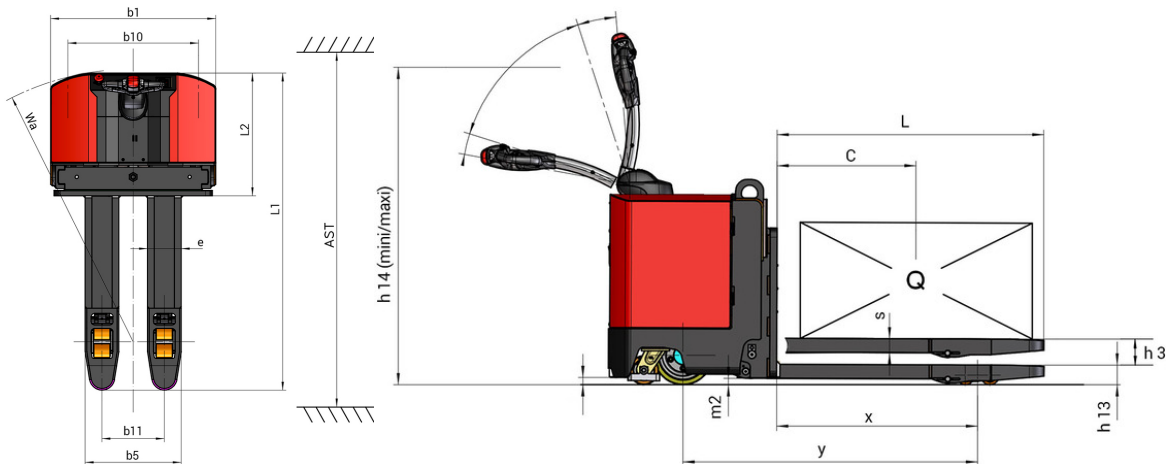
EP 740 - Disegno quotato
