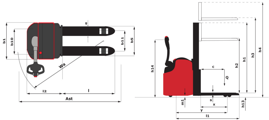
ES 730 - Disegno quotato
