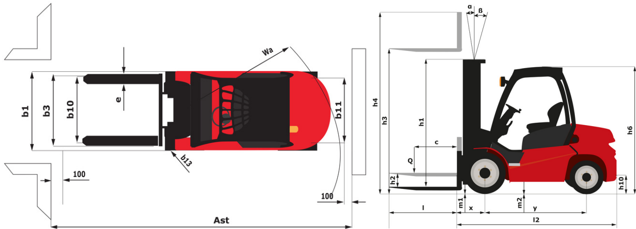
MI 15 G ST5 - Disegno quotato
