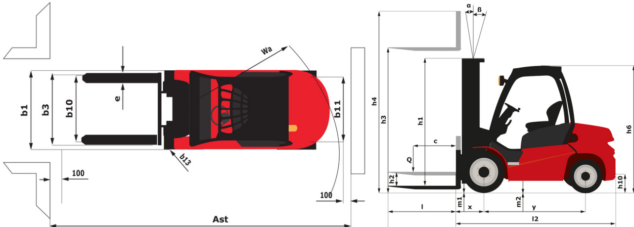
MI 20 D ST5 - Disegno quotato
