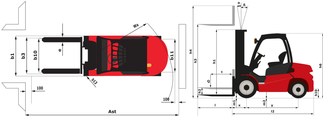
MI 50 D ST5 - Disegno quotato
