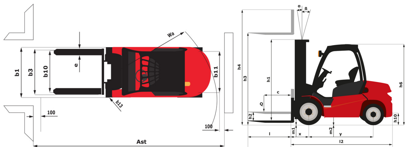
MI 50 LD ST5 - Disegno quotato
