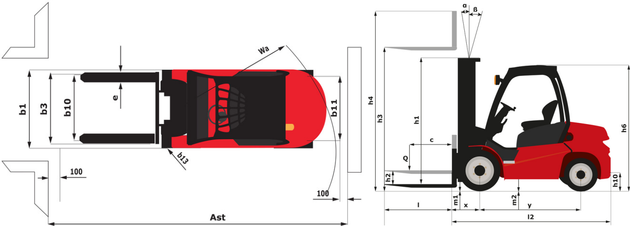
MI 60 D ST5 - Disegno quotato
