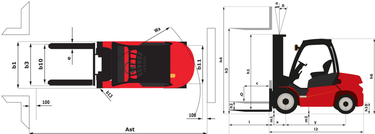
MI 80 D ST5 - Disegno quotato
