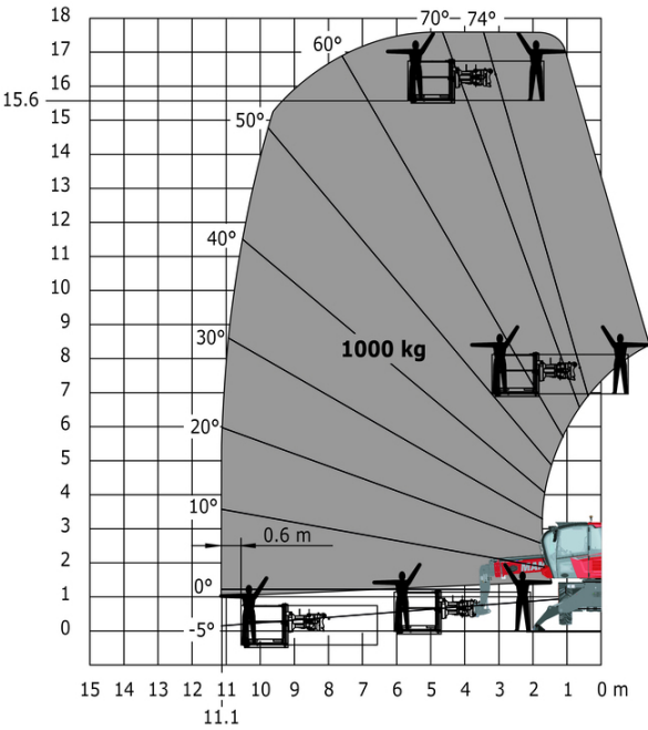
Rotazione su stabilizzatori con cestello da 1000 kg
