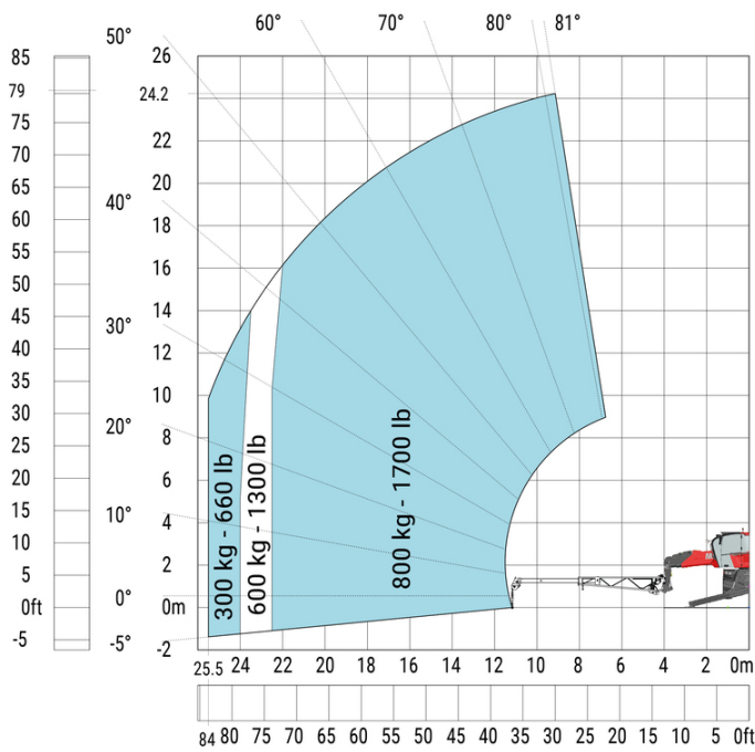
Macchina su stabilizzatori abbassati con braccio estensibile con verricello (metrico)
