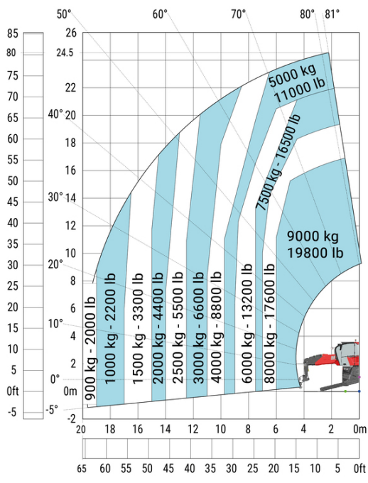
Macchina su stabilizzatori abbassati con gancio 9000 kg (metrico)
