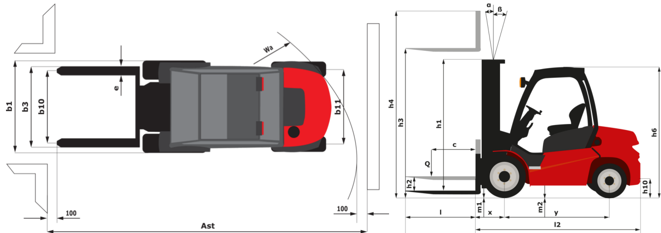
MSI 30 ST5 - Disegno quotato
