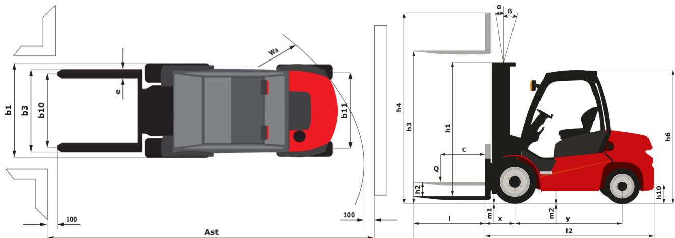
MSI 50 ST5 - Disegno quotato
